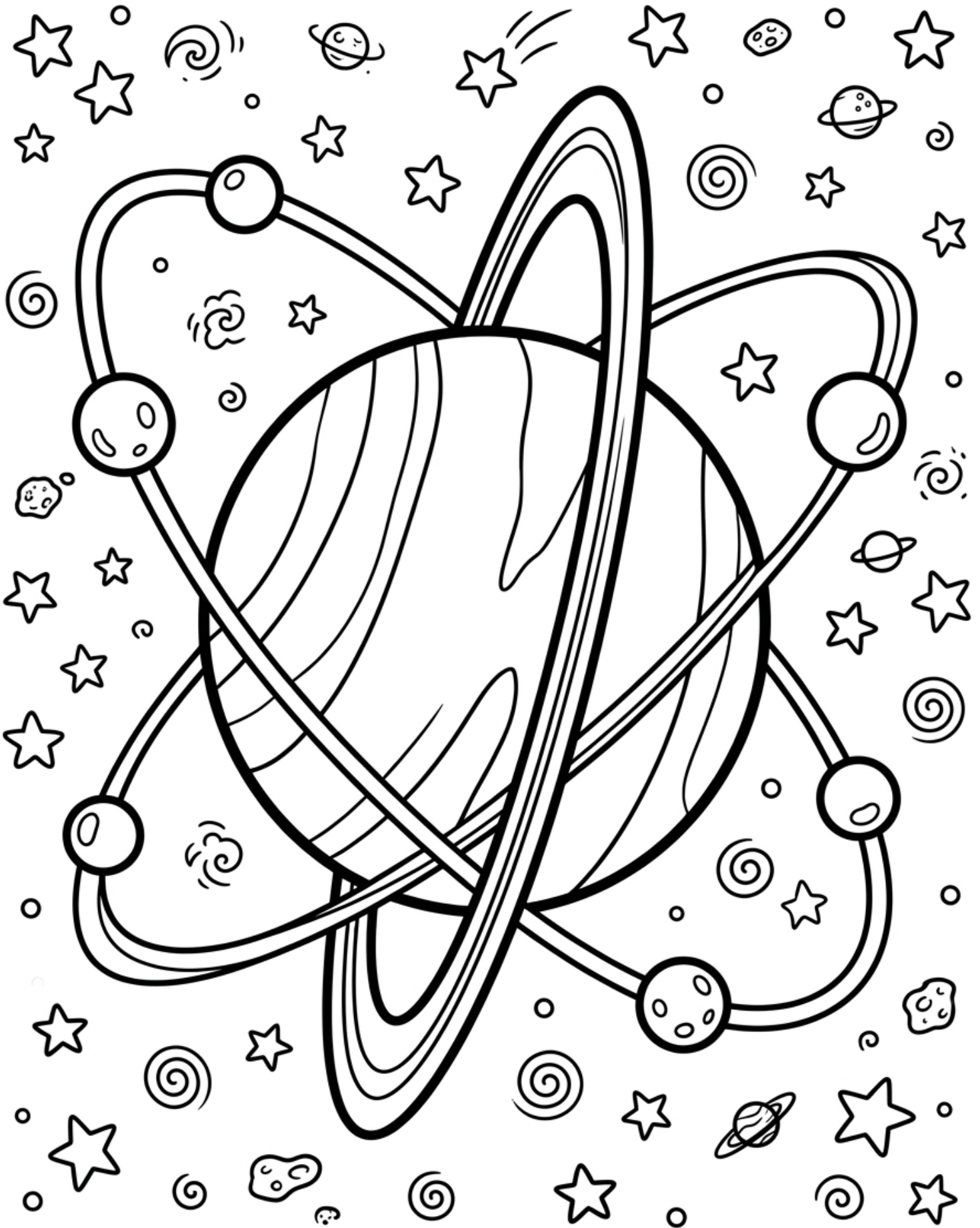
Uranus Tilt
